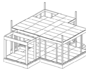
図1-3 2階床組
