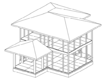
図1-4 小屋組
